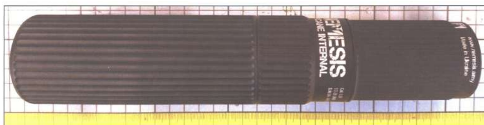
Зображення 1. Глушник звуку пострілу (саундмодератор) NEMESIS ARCANES INTERNAL.
